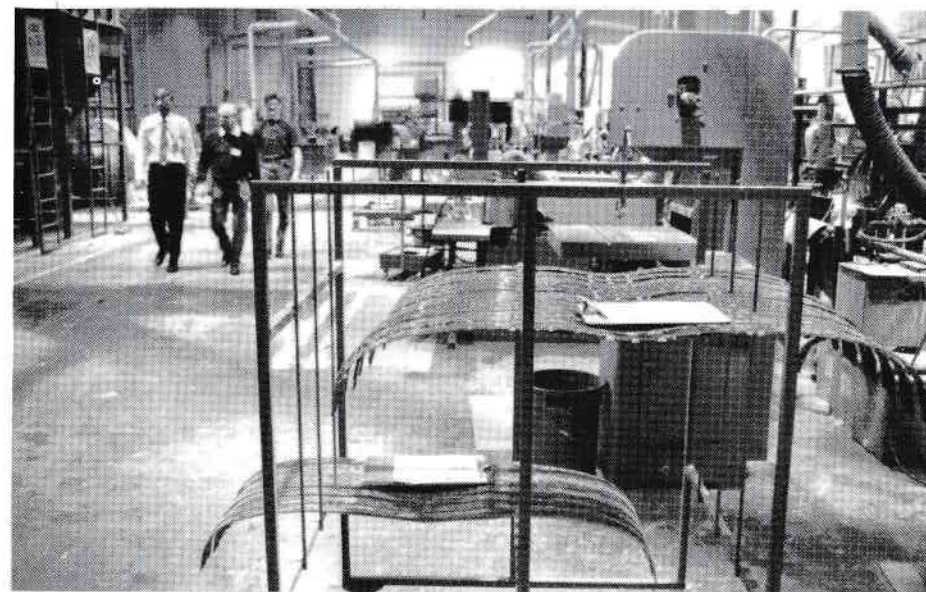
Lemtillverkning, närmast till compoundbågar, längre bort till rekurvbågar. Over och underlemmen hänger ihop tillsvidare.
