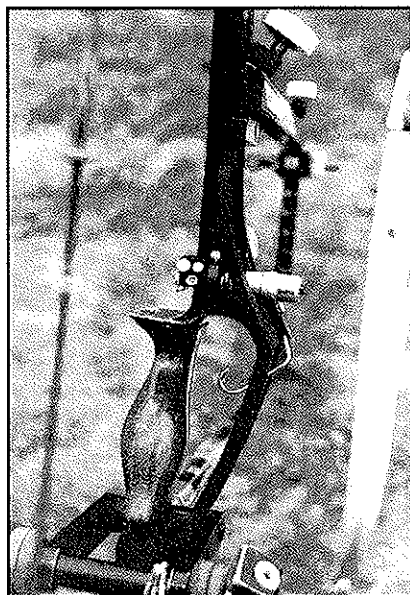
En bygel gör själva handtagssektionen styvare. Här ses en bild av Göran Bjerendals egen konstruktion.
