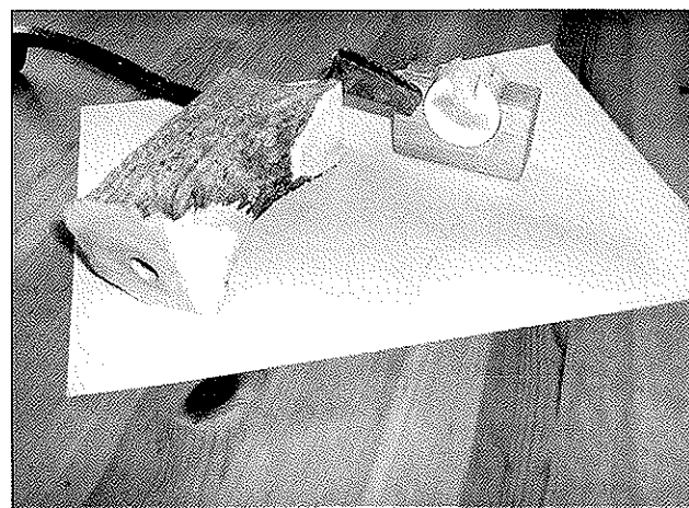
Här syns avtryckaren i svart smide och hur nöten i ben passar in i lagret av ek.
